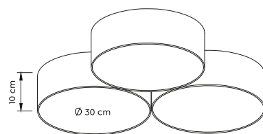
Deckenleuchte · Ceiling lamp ↔ 64,5 x 64,5 cm, ↑ 14 cm incl. SMD-LED, 38 W 4.200 lm, 3.000 K
