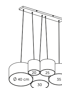
Pendelleuchte · Pendant ↔ 96,5 x 68,5 cm, ↓ 150 cm excl. 5 x E27, max. 42 W
