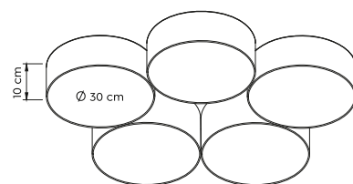
Deckenleuchte · Ceiling lamp ↔ 86,5 x 69 cm, ↑ 14 cm incl. SMD-LED, 58 W 6.300 lm, 3.000 K
